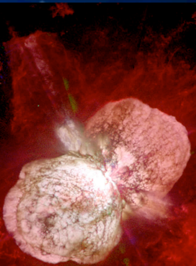
Eta Carinae
